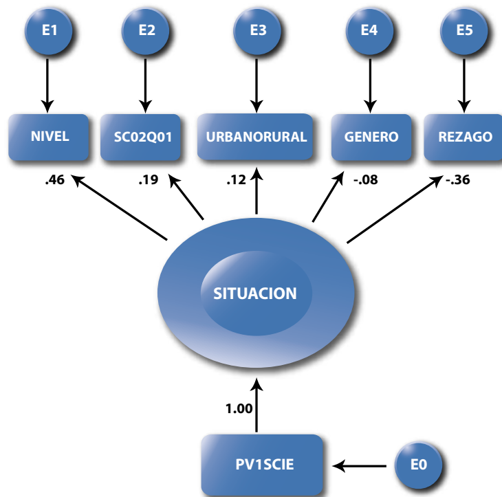
Figura A2.3 Modelo de ejemplo de ecuaciones estructurales
